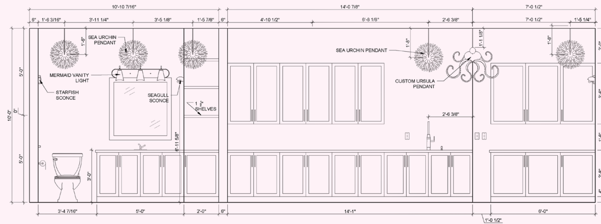
1 A5 - BATHROOM WEST WALL ELEVATION SCALE: 1/2" = 1'-0" 2 A5 - SNACK AREA WEST WALL ELEVATION SCALE: 1/2" = 1'-0"
