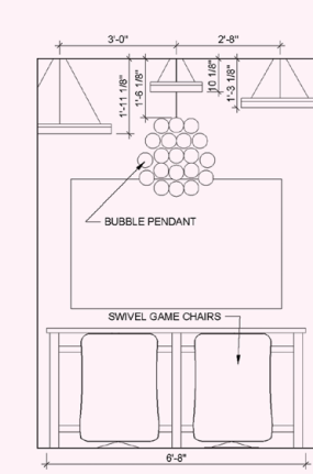
3 A7 - EAST WALL ELEVATION SCALE: 1/2" = 1'-0"
