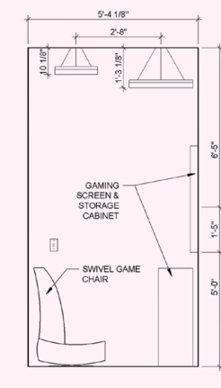
5 A7 - SOUTH WALL ELEVATION SCALE: 1/2" = 1'-0"
