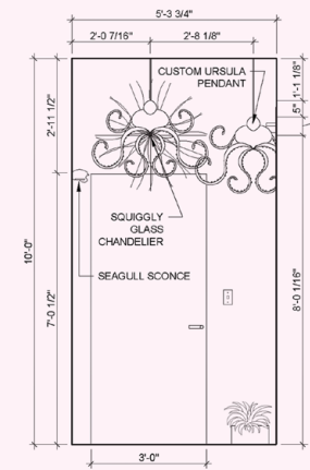
1 A7 - NORTH WALL ELEVATION SCALE: 1/2" = 1'-0"
